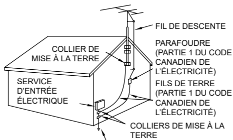
SYSTÈME DE MISE À LA TERRE DU RÉSEAU ÉLECTRIQUE (CODE CANADIEN DE L'ÉLECTRICITÉ)
